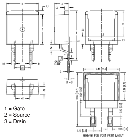
TO-263HV Outline
