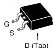
TO-263 (IXFA)
