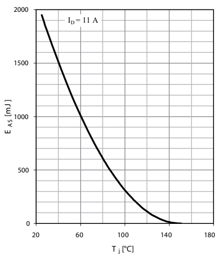
Fig. 9 Avalanche energy
