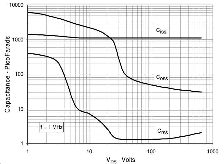
Fig. 12. Capacitance
