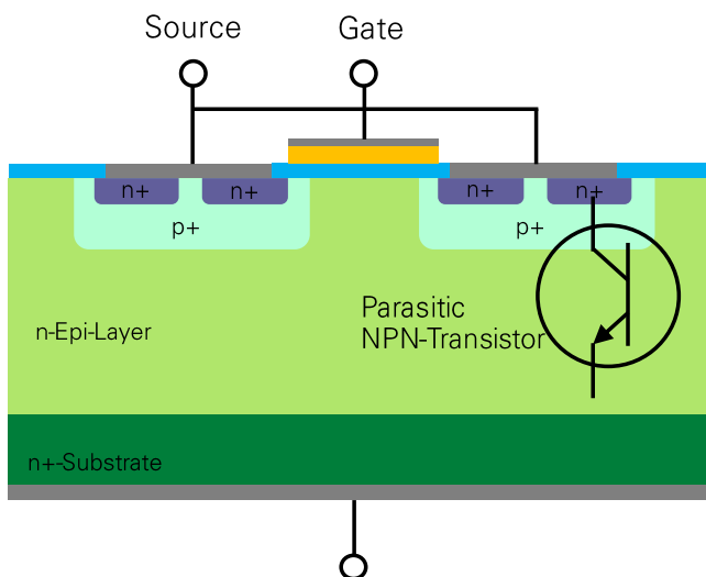
图 1. 包含寄生双极结晶体管(BJT)的 MOSFET 结构
