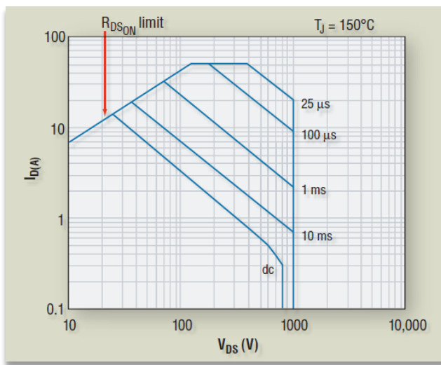
图 5. IXTK22N100L FBSOA 在 V_{DS} = 800 V、 I_D = 0.3 A、 T_C = 90^\circ C 时具有 240 W 功率耗散能力，以及其 SOA 工作点
