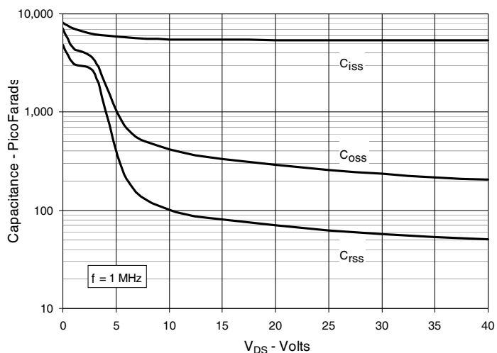
Fig. 12. Capacitance
